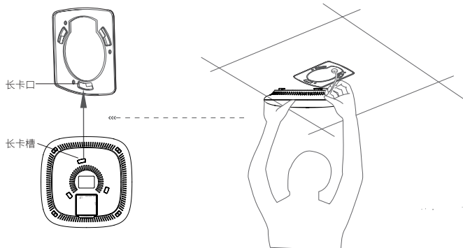
图3-5 安装AP到安装架示意图
